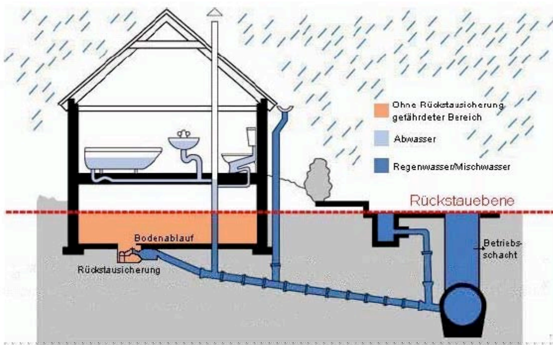
Sicherung gegen Rückstau Beispiel 1: Ausstattung aller Bodenabläufe mit einem "Rückstaudoppelverschluss"
